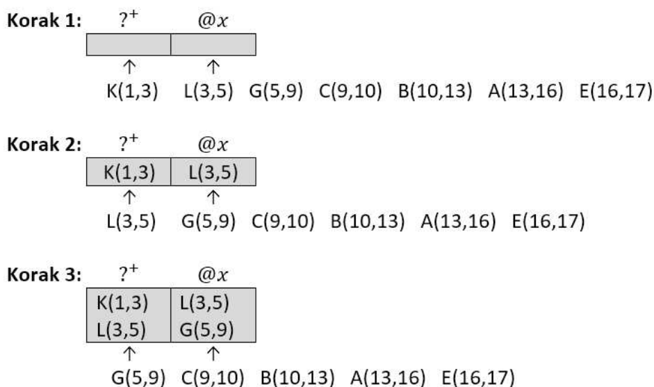
Slika 3.3: Primjer prva tri koraka kako IJP kreira listu za varijabilni predikat
