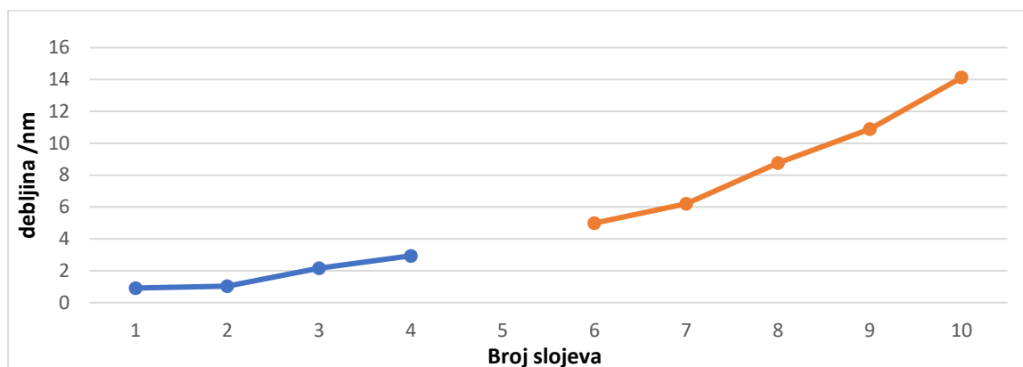
Slika 47. Debljina polielektrolitnih višeslojeva određena elipsometrijski korištenjem iterativne metode za svaki sloj adsorbiranog polielektrolita na Si/SiO 2 pločicu ( \theta = 25^\circ\text{C} ).
