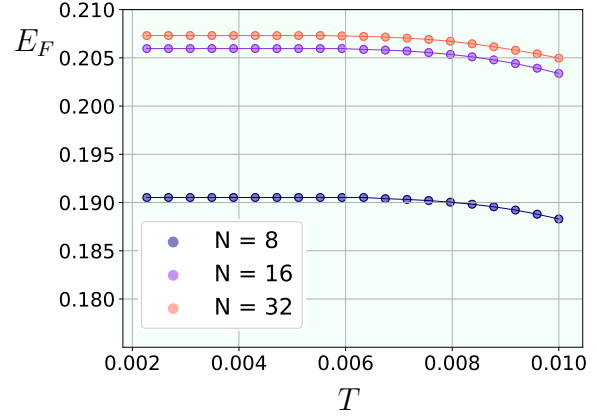
Slika 8.22: Negativnost \mathcal{N} (lijevo) i prepletenost formacije E_F (desno) kao funkcija temperature T , izračunato za Rydbergov model atoma u točki maksimalne prepletenosti \tilde{\Omega} = 0.05 za različite veličine sustava. Za negativnost: temperaturni raspon u kojem očekujemo točne rezultate označen je crvenom linijom za N = 16 i plavom linijom za N = 32 . Temperatura T izražena je u jedinicama J/k_B .
