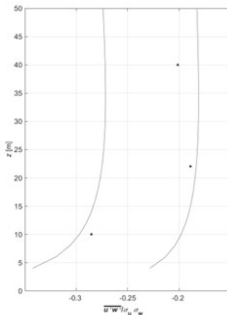
Slika 62: Vertikalni profil komponente Reynoldsovog smičnog naprezanja uspoređeni s vrijednostima iz ESDU 85020 (1985) za z_0=0,03 m uz raspon tolerancije \pm 20\% . Legenda: zvjezdica - usrednjena vrijednost promatranog \overline{u'w'}/\sigma_u\sigma_w , usrednjena kroz cijeli vremenski zapis za promatranu epizodu bure, siva krivulja - ESDU 85020 (1985).
