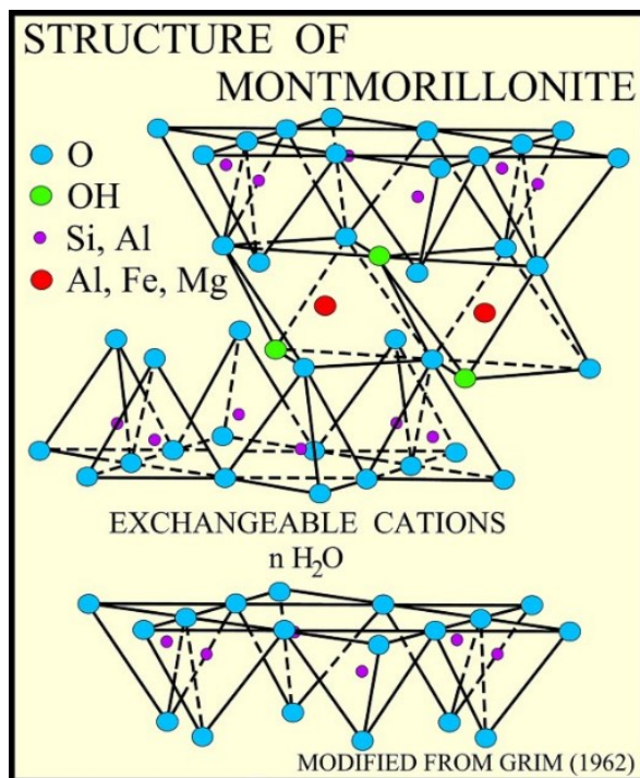
Slika 2: Struktura montmorillonita [2]
