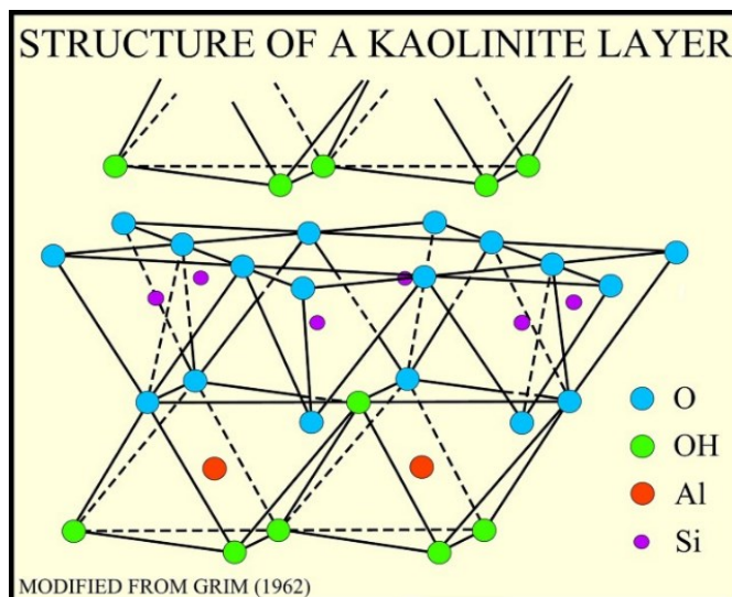
Slika 1: Struktura kaolinita [1]
