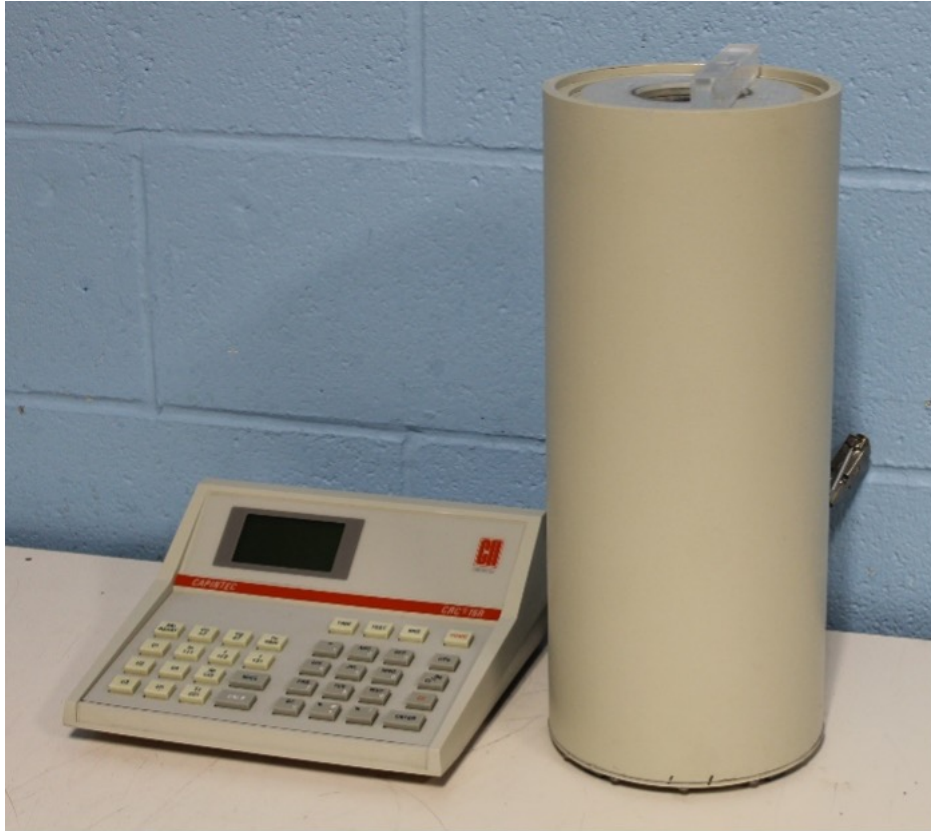
Slika 3.2: Mjerilo aktivnosti radioaktivnog uzorka Capintec 15R. (Slika je preuzeta iz [9].)
