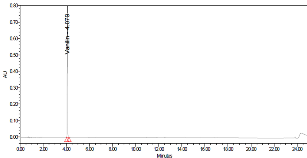
Slika 88. Kromatogram vanilina pri uvjetima Tg 42 i tg 23
