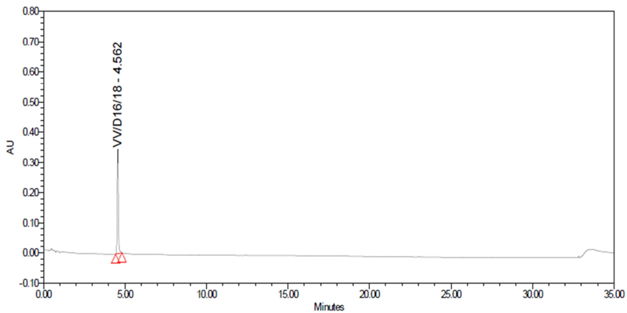
Slika 45. Kromatogram VV/D16/18 pri uvjetima Tg 30 i tg 30
