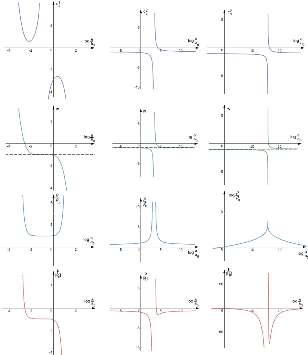
Slika 2.3: Grafički prikaz kozmičkih veličina u ovisnosti o parametrima i faktoru skale a . Prvi red: kvadrat brzine zvuka c_s^2 . Drugi red: parametar jednačbe stanja w . Treći red: gustoća energije normalizirana na današnju vrijednost \rho/\rho_0 . Četvrti red: tlak normaliziran na sadašnju apsolutnu vrijednosti p/|p_0| . Parametri: A = 1 i w_0 = -1.05 . Za lijevi stupac vrijedi B = -1/5 , za srednji stupac vrijedi B = 3/5 dok za desni stupac vrijedi B = 7/5 . Na svim grafovima os x je izražena u logaritamskoj skali, a os y u linearnoj, osim posljednjeg stupca za \rho(a) kod kojeg je i os y izražena u logaritamskoj skali kako bi se pokazala konačnost \rho u a_* .
