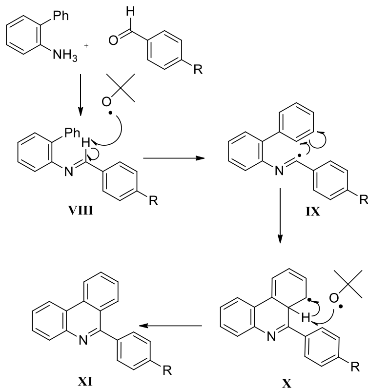
Shema 3. Mehanizam radikalne homolitičke aromatske supstitucije pri sintezi 6-arilfenantridina iz diariliminskih prekursora.
