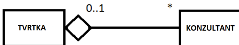
Slika 3.2: Agregacija
