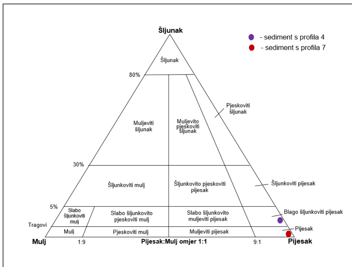
Slika 4.2. Trokomponentni dijagram uzoraka sedimenta s profila 4 i 7 plaže Sakarun.
