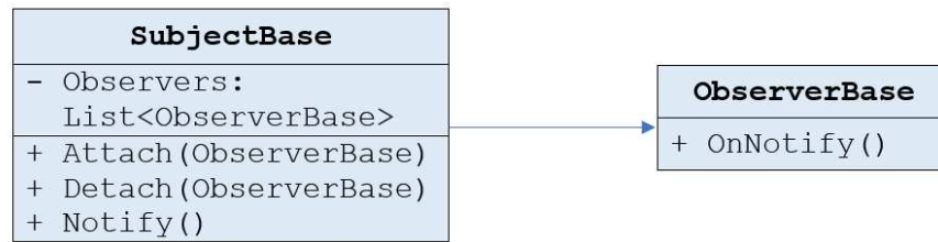
Slika 2.3: Observer Pattern
