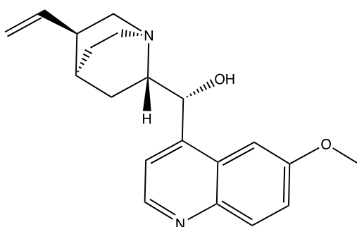
Slika 20. Strukturna formula kinina.
