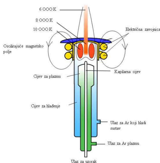
Slika 5. Shematski prikaz nastajanja induktivno spregnute plazme. Preuzeto i prilagođeno iz literaturnog izvora 20 .
