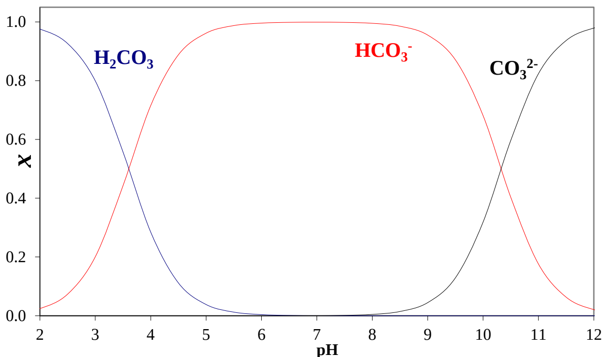
Slika 3. Dijagram specijacija ugljične kiseline pri temperaturi od 273,15 K.
