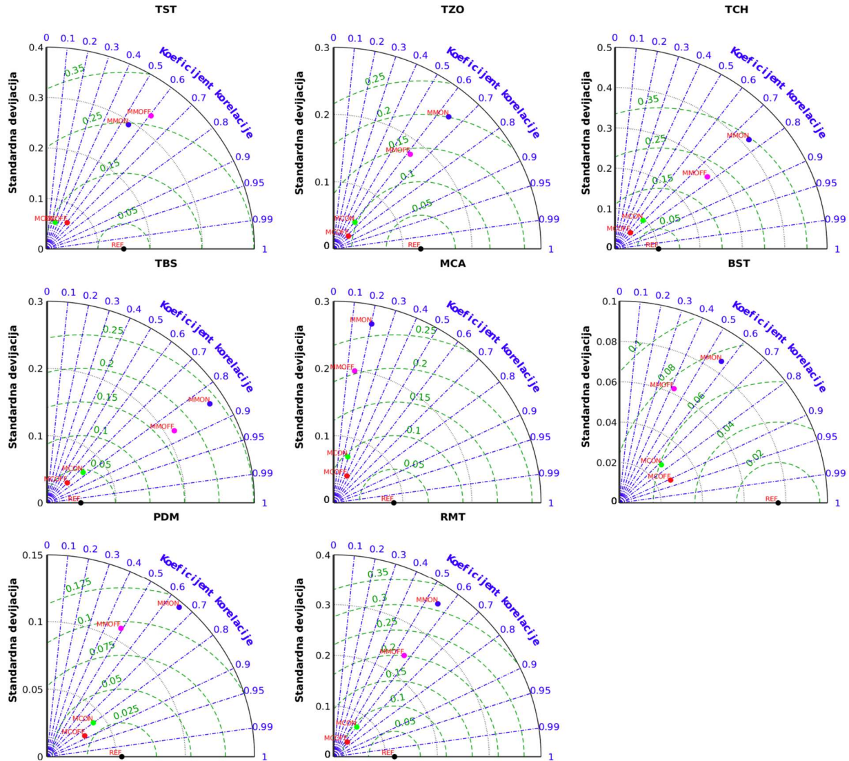
Slika 34. Taylorov dijagram za parametar AOD, mjereno na osam postaja (Tablica 2b) (crna točka) i simuliran s četiri različita postava modela (Tablica 5): MCON (zelena točka), MCOFF (crvena točka), MMON (plava točka) i MMOFF (roza točka). Standardna devijacija je predstavljena crnom točkastom, koeficijent korelacije plavom, a RMSD sa zelenom isprekidanom linijom.
