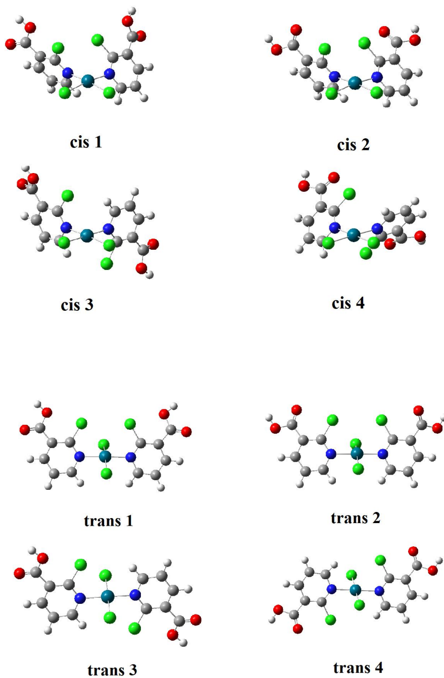
Slika 20. Optimizirane geometrije trans i cis izomera [\text{PdCl}_2(2\text{-ClnicH})_2] .
