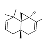
tujopsen
