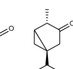
\alpha -tujon
