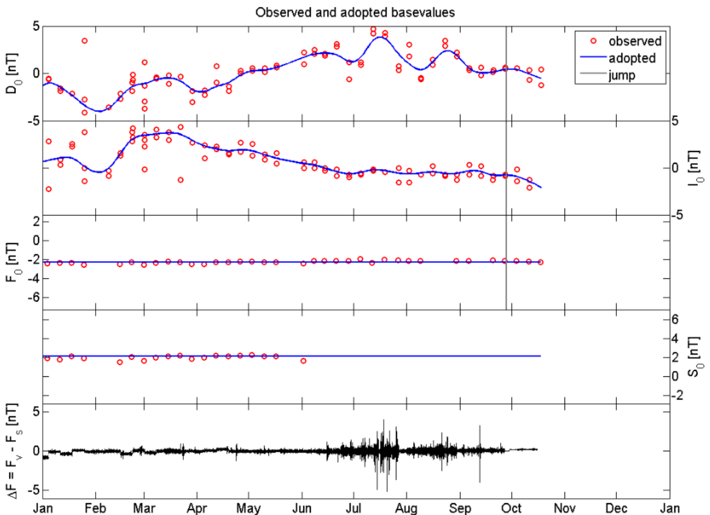
Slika 2.2 – Opažene ( engl. observed ) i prilagođene ( engl. adopted ) kalibracijske vrijednosti za DIDD variometar. Na slici su također prikazani rezultati motrenja s početka listopada koji su korišteni u izračunu kalibracijskih krivulja za rujan.
