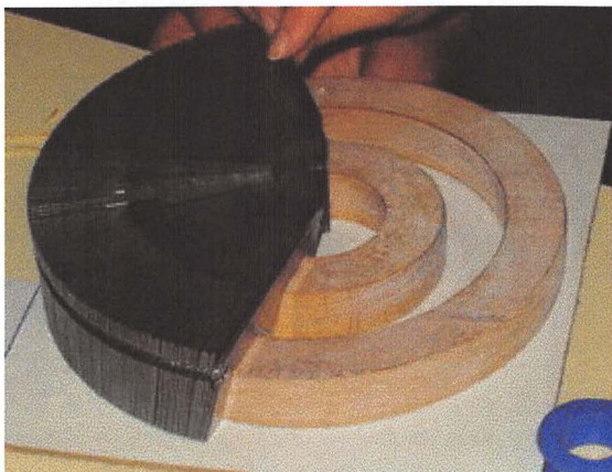
Slika 9a. Lepezasto složeni limovi
