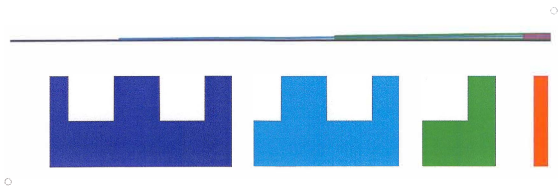
Slika 8a. Oblik transformatorskih limova i način slaganja
