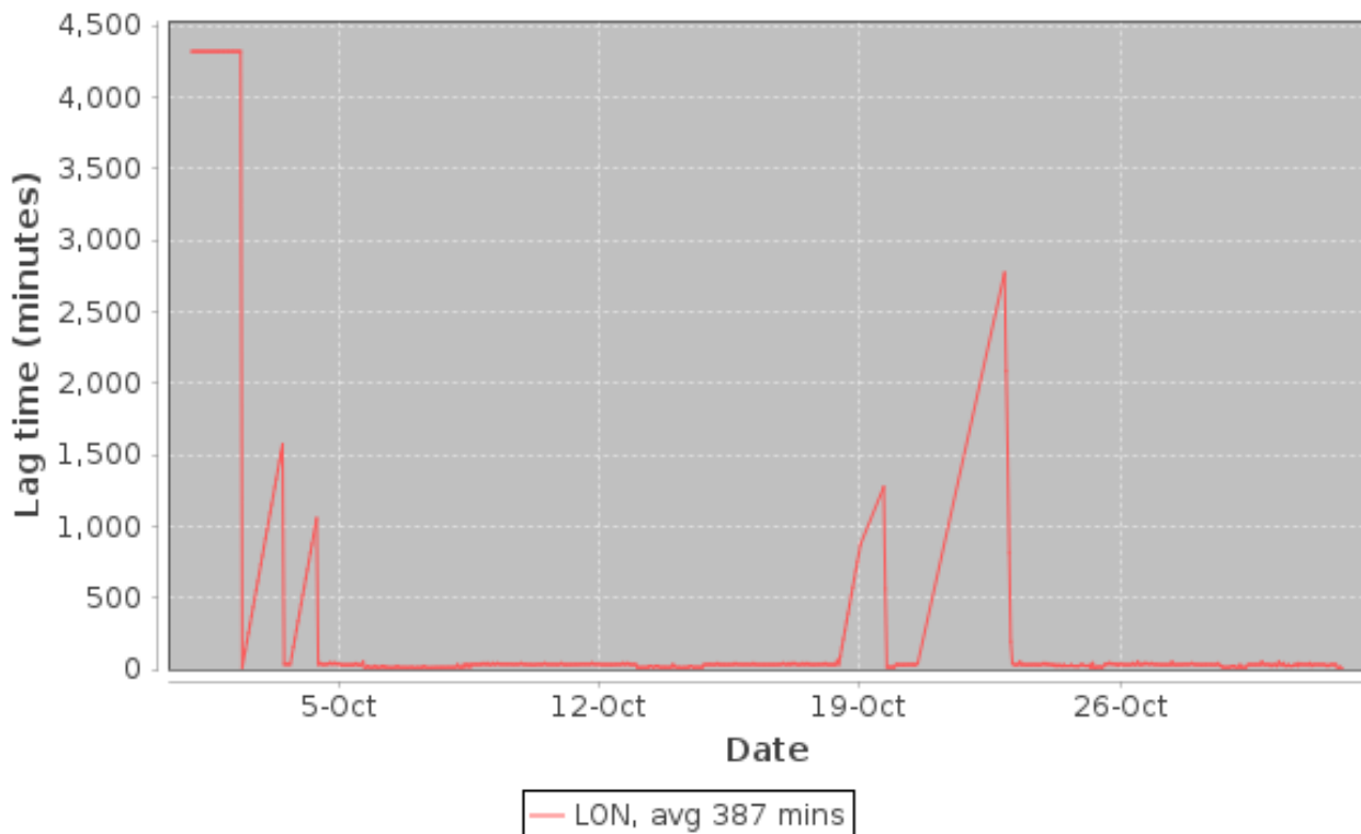
Slika 2.1 – Kašnjenje u dostupnosti podataka u realnom vremenu, listopad 2023.
