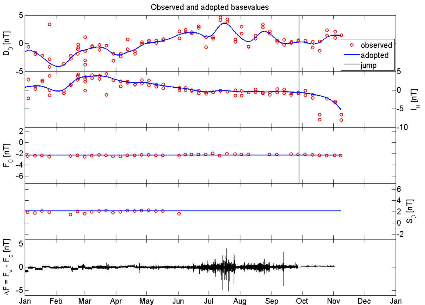
Slika 2.2 – Opažene ( engl. observed ) i prilagođene ( engl. adopted ) kalibracijske vrijednosti za DIDD variometar. Na slici su također prikazani rezultati motrenja s početka studenog koji su korišteni u izračunu kalibracijskih krivulja za listopad.
