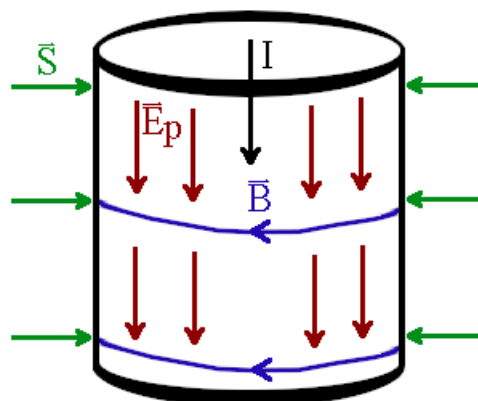
Slika 4.4: Žicu blizu žarulje modeliramo cilindrom radijusa r i visinom d . Na slici označeni su smjer struje I , magnetsko polje na površini vodiča B , smjer električnog polja E na površini vodiča i Poyntingov vektor S .
