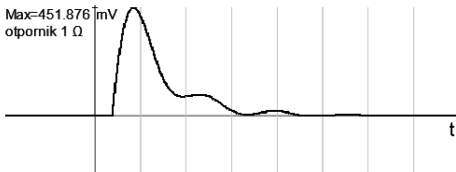
Slika 4.18: Rezultati za napon na otporniku otpora R = 1 \Omega u slučaju da strujni krug nije zatvoren.
