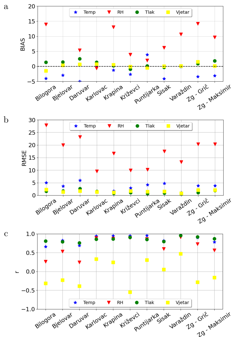
Slika 3.10. Statističke veličine 2. lipnja 2022. - (a) pristranost (BIAS), (b) korijen srednje kvadratne pogreške (RMSE), (c) koeficijent korelacije ( r ) za temperaturu zraka (plavo), relativnu vlagu (crveno), tlak zraka (zeleno) i brzinu vjetra (žuto) za odabrane postaje.
