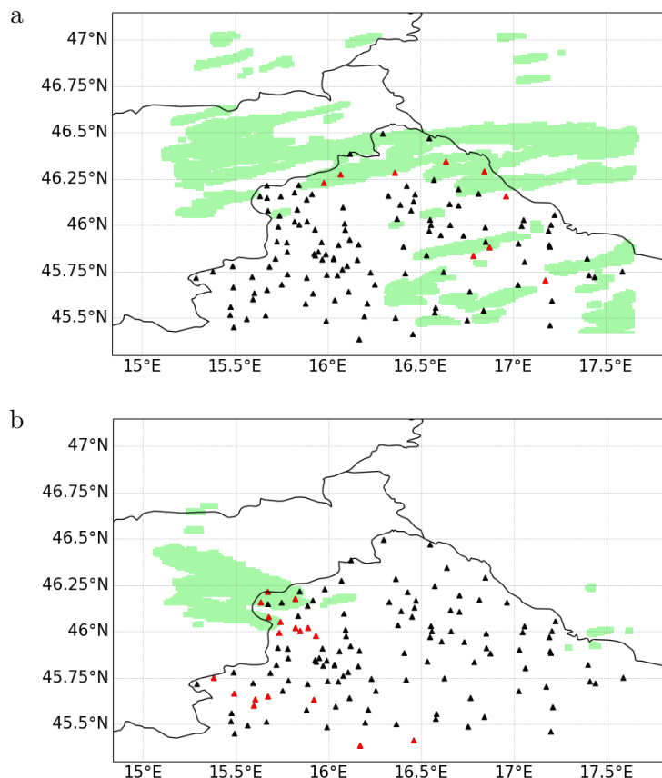
Slika 3.12. Simulirani trag tuče unutar 24 sata i mreža DHMZ-ovim prizemnih postaja za (a) 25. svibnja 2022. i (b) 2. lipnja 2022. Crni trokutići označavaju postaje na kojima nije bilo tuče, a crvene one na kojima je tuća opažena.
