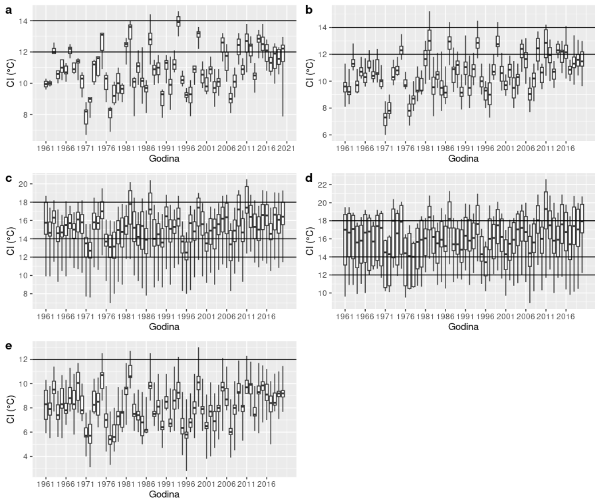
Slika 4.4 a) Kutijasti dijagrami za CI (°C) izračunatog za 80 meteoroloških postaja u razdoblju 1961.-2020. podijeljenih po vinogradarskim regijama u Hrvatskoj; (a) Slavonija i Hrvatsko Podunavlje (zona C I), (b) Središnja bregovita Hrvatska (zona B), (c) Hrvatska Istra i Kvarner (zona C II), (d) Dalmacija (zona C II i C III), (e) planinski dio Hrvatske. Linije kutijastih dijagrama označavaju medijane, gornji i donji dio okvira prikazuju 75. i 25. percentil. Horizontalne linije označavaju klase CI (vidi Tablicu 3.1).
