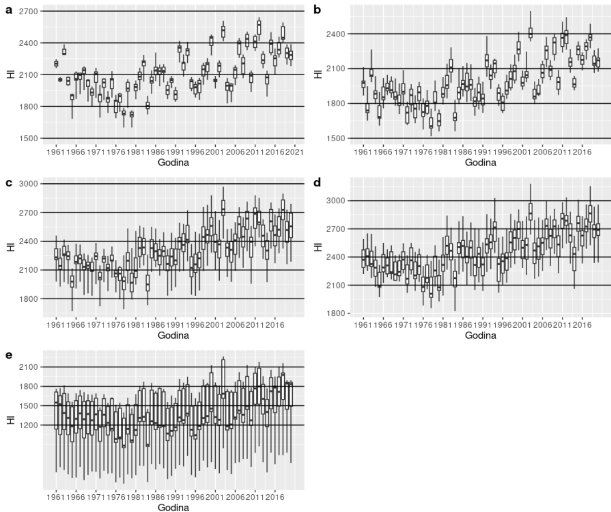
Slika 4.3 Kutijasti dijagrami za indeks HI (°C jedinice) izračunat za 80 meteoroloških postaja u razdoblju 1961.-2020. podijeljenih po vinogradarskim regijama u Hrvatskoj; (a) Slavonija i Hrvatsko Podunavlje (zona C I), (b) Središnja bregovita Hrvatska (zona B), (c) Hrvatska Istra i Kvarner (zona C II), (d) Dalmacija (zona C II i C III), (e) planinski dio Hrvatske. Linije kutijastih dijagrama označavaju medijane, gornji i donji dio okvira prikazuju 75. i 25. percentil. Horizontalne linije označavaju klase HI (vidi Tablicu 3.1).
