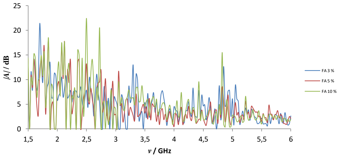
Slika 79. Ovisnost apsolutne vrijednosti apsorpcije ( |A| ) za dvokomponente glinene kompozitne materijale s različitim udjelima lebdećeg pepela (FA) o frekvenciji ( \nu ).
