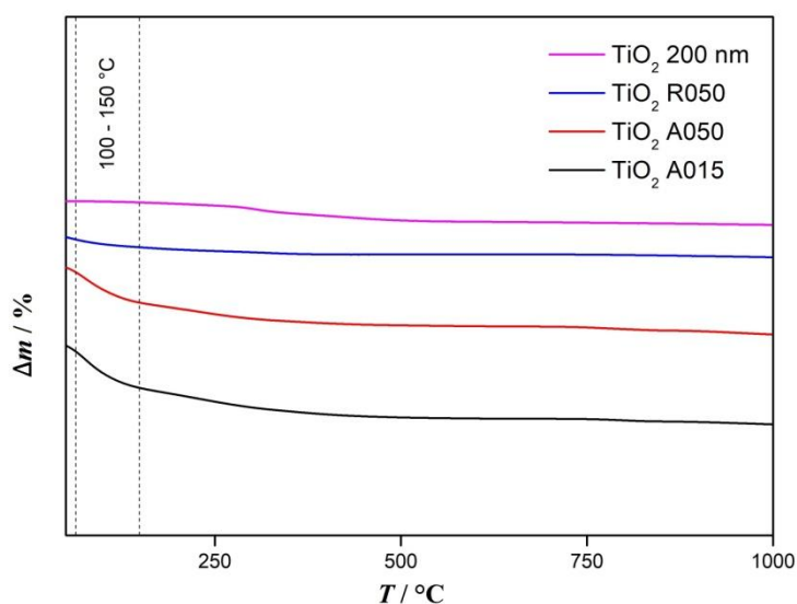
Slika 29. Termogravimetrijska krivulja ovisnosti gubitka mase o temperaturi četiri različita uzorka titanijevog dioksida pri čemu je: \text{TiO}_2 200 nm rutil veličine čestica 200 nm, \text{TiO}_2 R050 je rutil veličine čestica 50 nm, \text{TiO}_2 A050 anatas veličine 50 nm i \text{TiO}_2 A015 je anatas veličine čestica 15 nm.
