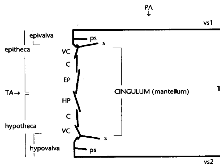
Slika 1. Struktura frustule
