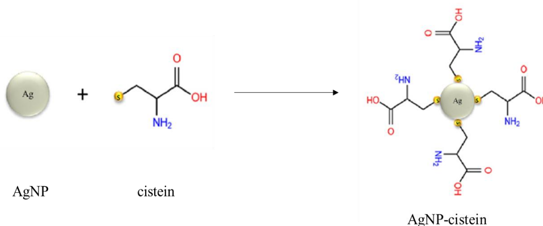
Slika 9. Shematski prikaz stvaranja Ag-sulfhidrilne veze između AgNP i molekula cisteina. Preuzeto i prilagođeno prema Bamdad i sur. (2016).
