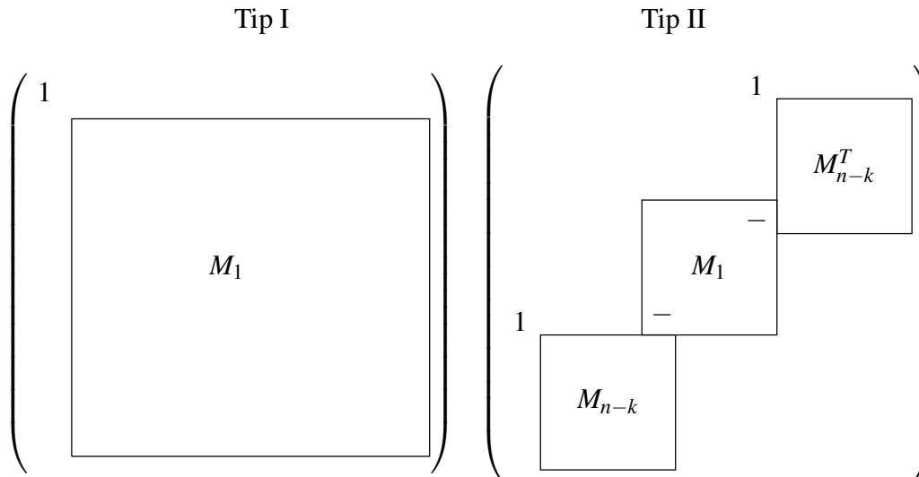
Slika 2.12: Dva tipa \mathcal{C}_{\mathcal{D}} -matrica reda n + 1 .
