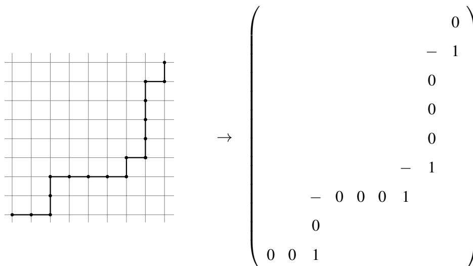
Slika 3.6: 1-ice pridružene vrhovima i -1 -ice pridružene dolinama Dyckovog puta.
