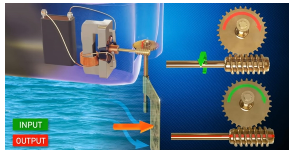
Slika 2.4: Mehanizam pužnog prijenosa
