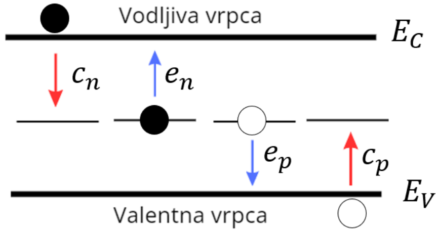
Slika 2.2: Shematski prikaz uhvata i emisije elektrona i šupljina. Označene su energije vodljive vrpce E_C i valentne vrpce E_V te vjerojatnost uhvata elektrona c_n , vjerojatnost emisije elektrona e_n , vjerojatnost emisije šupljine e_p i vjerojatnost uhvata šupljine c_p .
