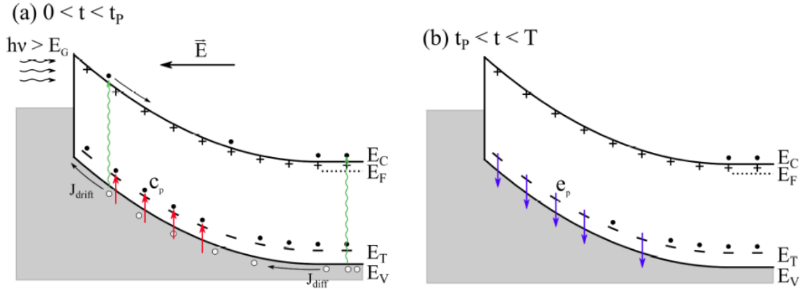
Slika 3.5: Shematski prikaz procesa dobivanja MCTS signala. a) Uхват šupljina iz valentne vrpce u duboke nivoe tijekom primjene svjetlosnih pulseva. b) Emisija šupljina iz dubokih nivoe nakon svjetlosnog pulsa. Slika preuzeta iz literature [26].
