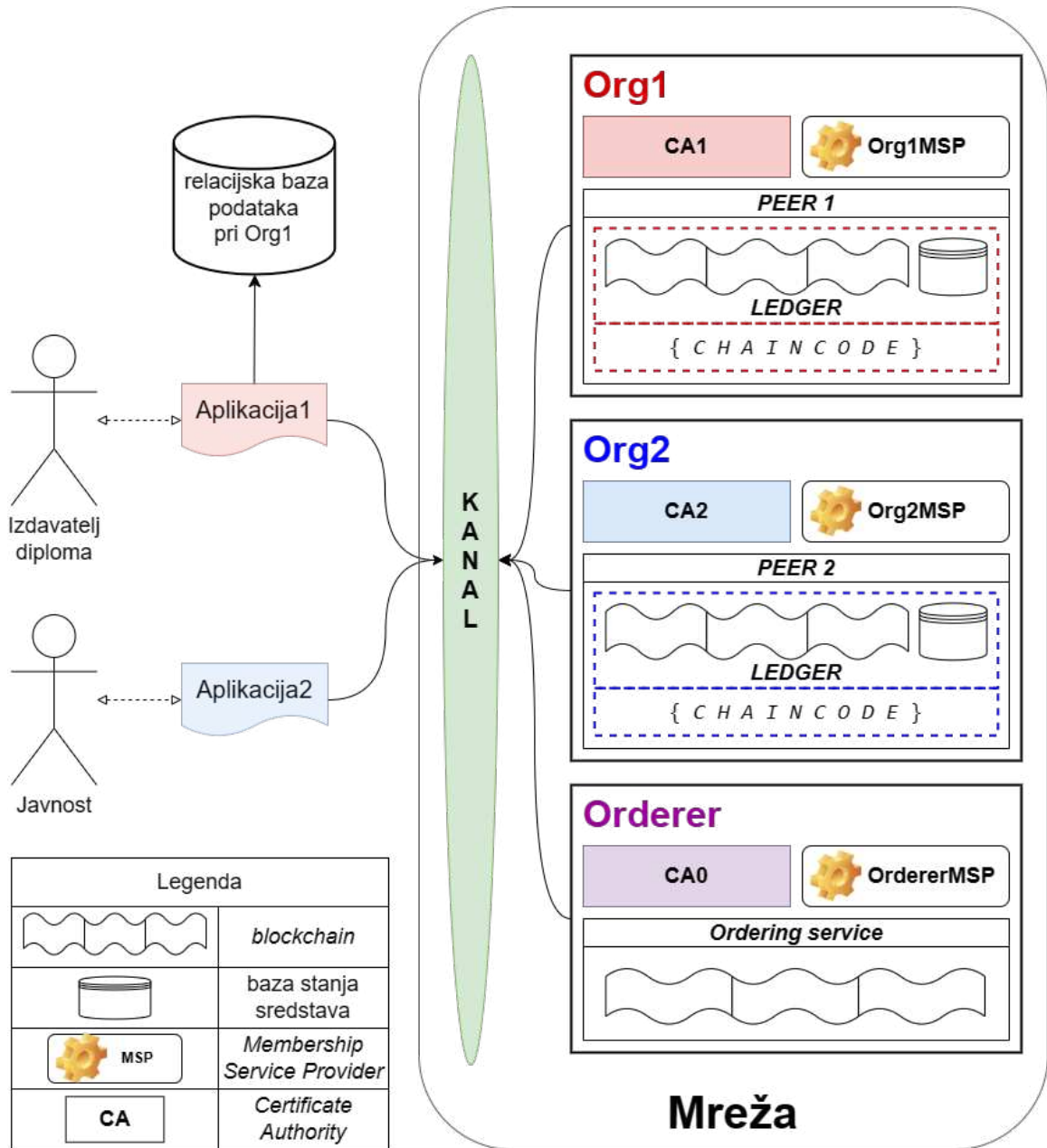
Slika 3.1: Shema sustava
