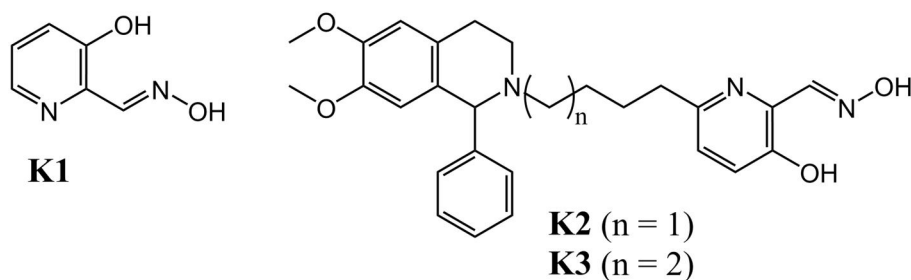
Slika 24. Konjugati fenil-tetrahidrozokinolina i piridinaldoksima. 109
