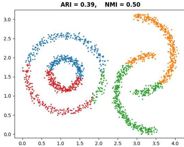
Slika 4.3: Particioniranje metodom k - sredina
