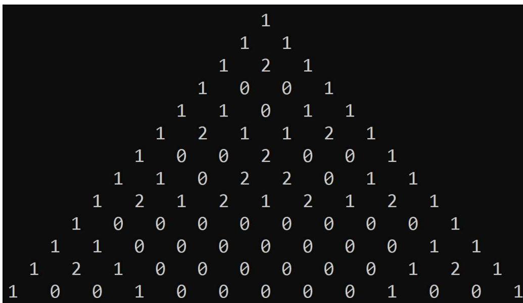
Slika 3.5: Pascalov trokut modulo 3
