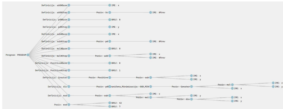
Slika 2.3: Stablo parsiranja
