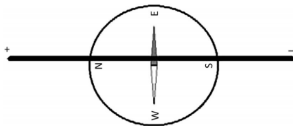
Slika 3. Oerstedov eksperiment, vodič je prvo smješten ispod kompasa, a zatim je puštena struja [19]
