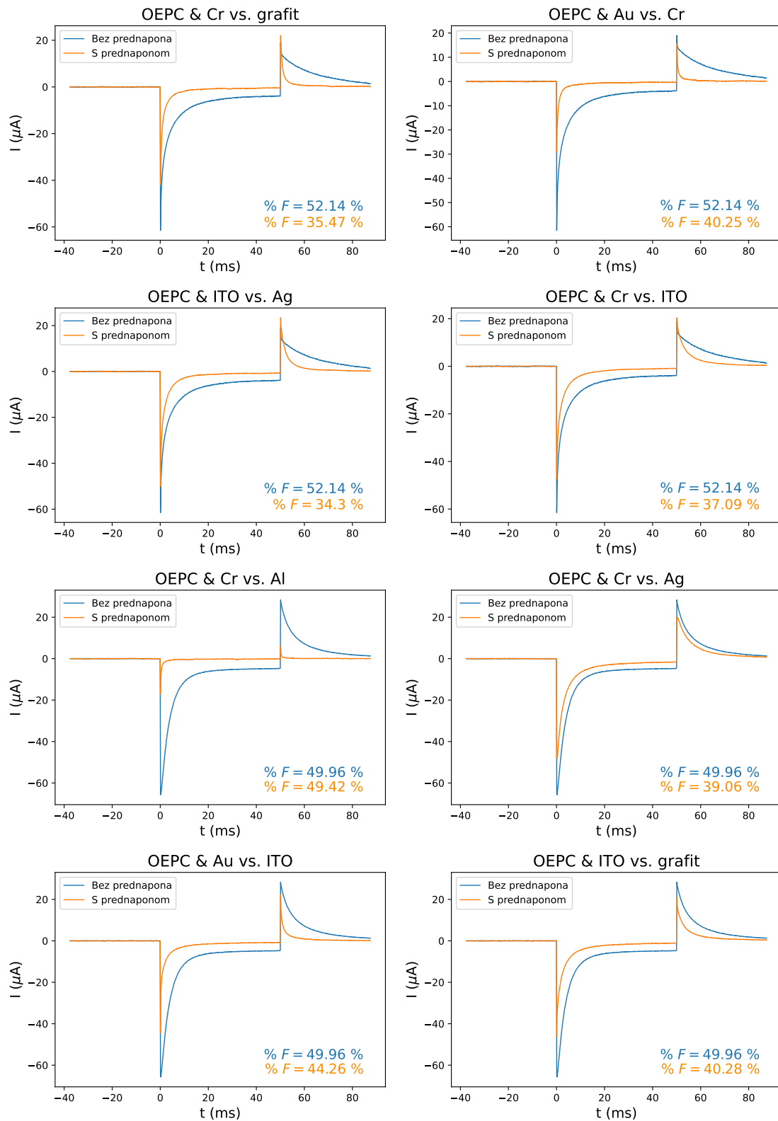
Slika 7.15: Fotostruja fotokondenzatora za uzorak bez prednapona (plavo) i s galvaniskim prednaponom (narančasto). Odgovarajuće vrijednosti \%F su označene na grafovima istim bojama kao i krivulje.
