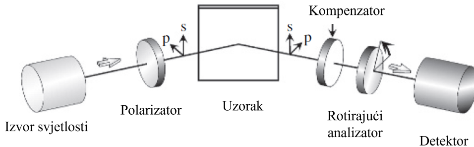
Slika 6.4: Shematski prikaz elipsometra sa rotirajućim analizatorom i kompensatorom. Preuzeto i prilagođeno iz [45].
