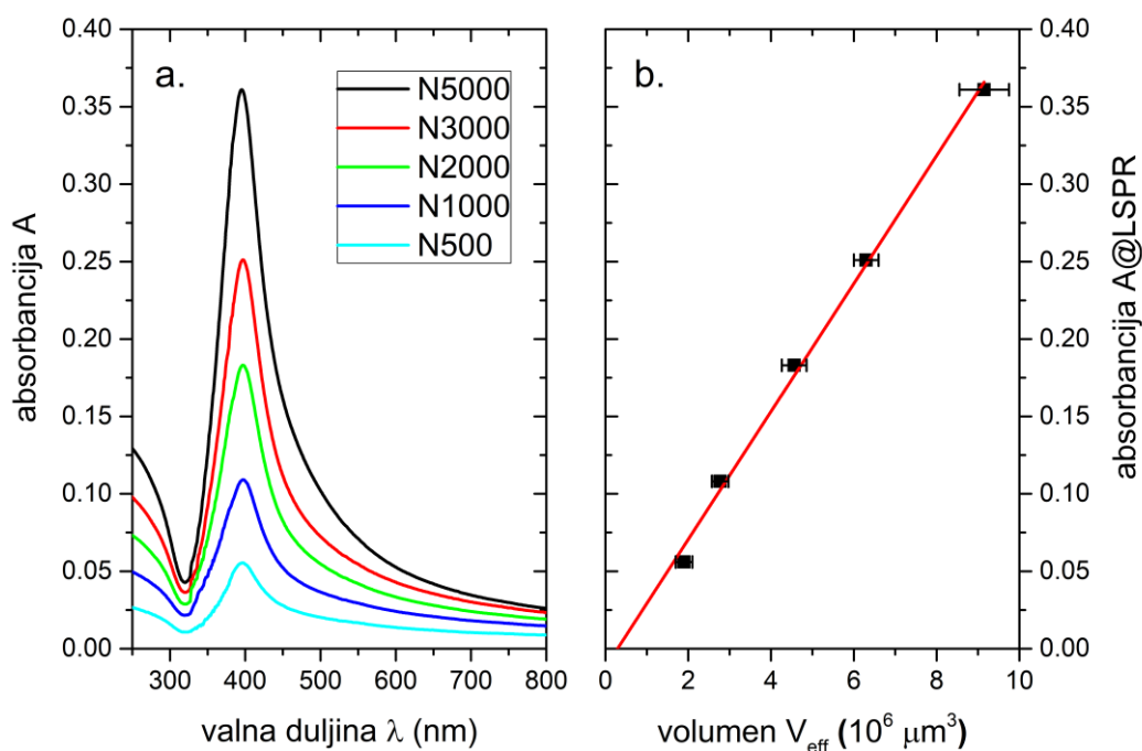
Slika 44. Ovisnost absorbancije o valnoj duljini ulazne svjetlosti za kraterе ablatirane sa različitim brojem laserskih pulseva (a.) i ovisnost absorbancije na LSPR-u o efektivnom volumenu kratera za pripadni broj laserskih pulseva (b.).
