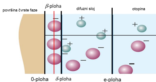
Slika 6. Shematski prikaz Gouy-Chapman-Sternova (GCS) modela s naznačenim ploham i karakterističnim makroskopskim područjima. Radi jasnoće prikaza, \beta -ploha je označena crvenom punom crtom. Površina metalnog oksida/koloidne čestice je pozitivno nabijena.
