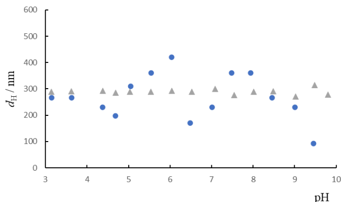
Slika 20. pH ovisnost hidrodinamičkog promjera koloidnih čestica \text{SiO}_2 (●) i uz dodan P4VP polielektrolit ( c(\text{P4VP}) = 1 \times 10^{-4} \text{ mol dm}^{-3} ) (▲) pri 25^\circ\text{C} . Ionska jakost koloidne suspenzije iznosila je I_c = 2 \times 10^{-3} \text{ mol dm}^{-3} ; \gamma(\text{SiO}_2, \text{s}) = 5 \text{ g dm}^{-3} .
