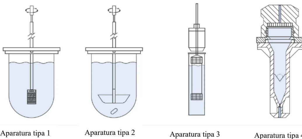
Slika 2.10. Shematski prikazi aparatura za oslobađanje djelatnih tvari 64
