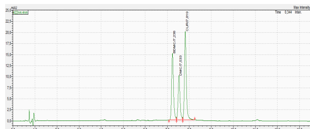
Slika 8.17. Kromatogrami kurkuminoida i piperina u uzorku DP 17 nakon 120 minuta oslobađanja u (a) SDS, (b) FaSSGF, (c) FeSSIF i (d) FaSSIF mediju
