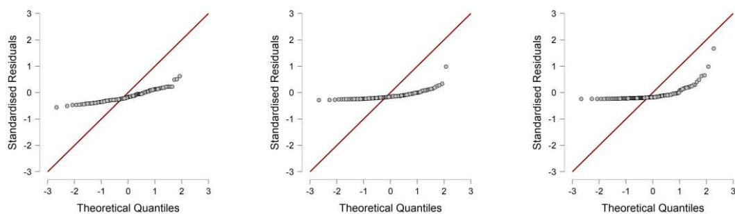
Slika 44. QQ-plot odstupanja.
