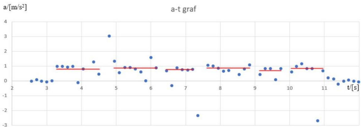
Slika 14 - Graf akceleracije nacrtan u Excelu pomoću podataka u csv datoteci, crvene linije označavaju prosječnu vrijednost akceleracije u tom vremenskom intervalu, prikazane vrijednosti su 0.78 \text{ m/s}^2 , 0.83 \text{ m/s}^2 , 0.76 \text{ m/s}^2 , 0.84 \text{ m/s}^2 , 0.74 \text{ m/s}^2 , te 0.84 \text{ m/s}^2
