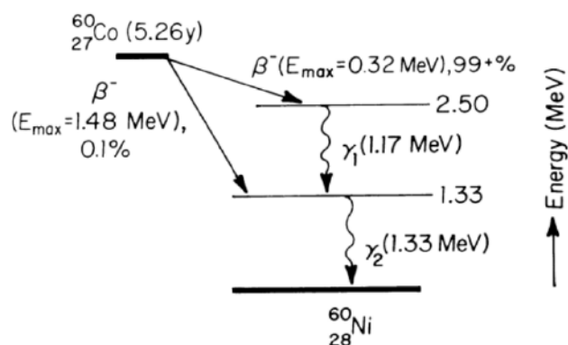
Slika 3.2: Dijagram radioaktivnog raspada ^{60}\text{Co} [4].
