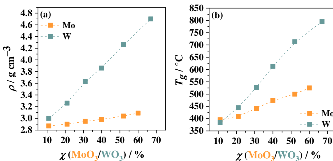
Slika 35. Ovisnost (a) gustoće, \rho , i (b) staklišta, T_g , o udjelu MoO_3 odnosno WO_3 za stakla iz serije 2: \chi MoO_3 - (60 - \chi) V_2O_5 - 40 P_2O_5 , \chi = 11 - 60 % i serije 3: \chi WO_3 - (60 - \chi) V_2O_5 - 40 P_2O_5 , \chi = 11 - 67 %.
