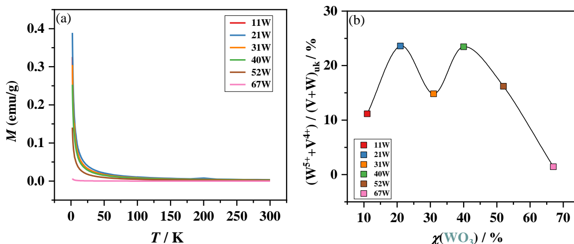
Slika 39. (a) Krivulje temperaturne ovisnosti magnetizacije, M(T) , i (b) omjer (W^{5+} + V^{4+}) / (V + W)_{\text{uk}} u ovisnosti o udjelu \text{WO}_3 za stakla iz serije 3 : \chi\text{WO}_3 - (60 - \chi)\text{V}_2\text{O}_5 - 40\text{P}_2\text{O}_5 , \chi = 11 - 67 %.
