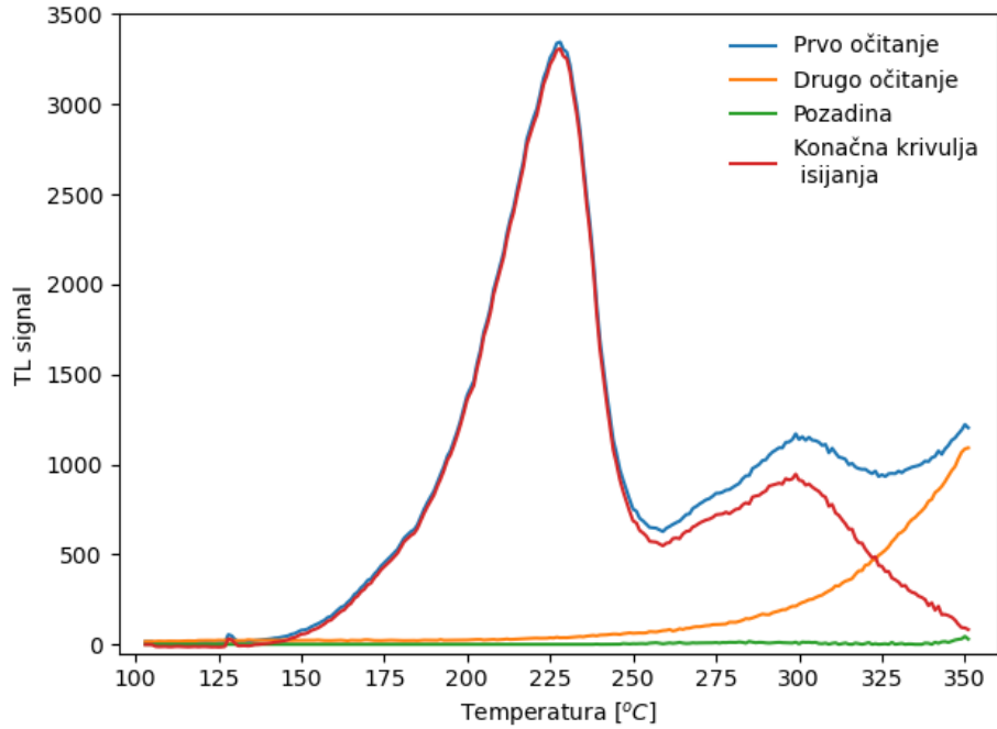
Slika 3.11: Prikaz dobivanja konačne krivulje isijanja dozimetra zračenog protonima energije 5 MeV. Ona se dobije oduzimanjem intrinzičnog signala (drugo očitanje) i pozadine od ukupnog signala ozračenog dozimetra (prvo očitanje).
