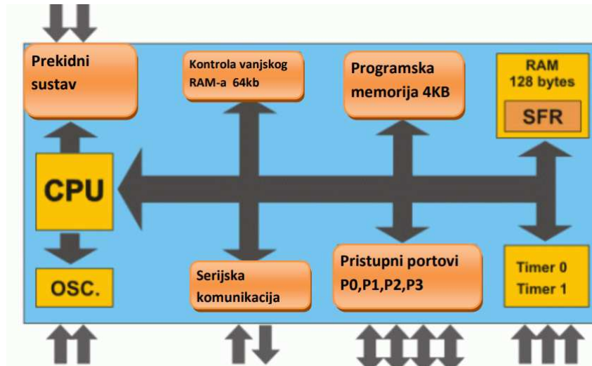
Slika 2.5: Unutrašnjost mikrokontrolera
