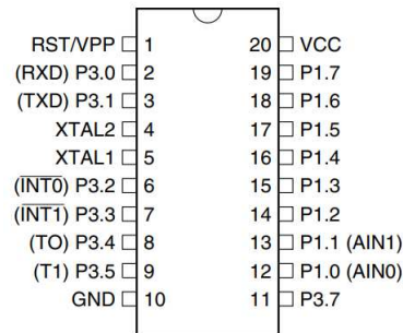
Slika 2.4: Mikrokontroler AT89C4051
