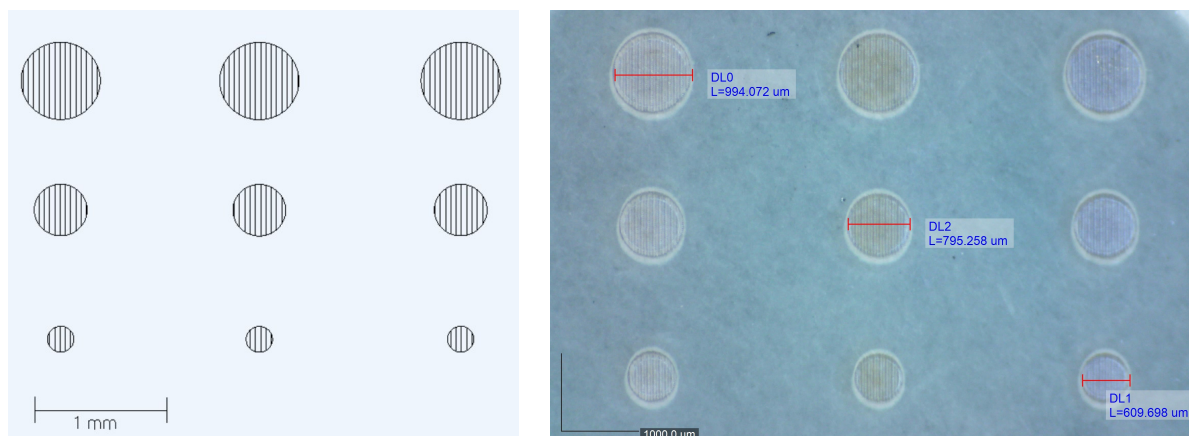
Slika 6.33: Lijevo: Dizajn uzorka za strukturiranje OEPC-a iz LMS programa. Desno: Proizvedeni uzorak na OEPC-u gdje su stupci proizvedeni s 16%, 14% i 15% postavkom atenuatora i možemo jasno vidjeti razlike u bojama donjeg sloja.
