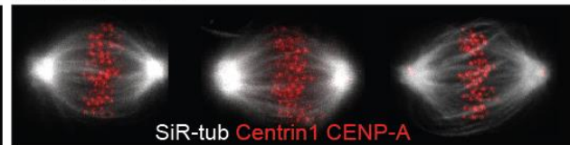
MG-132
