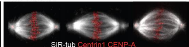
HAUS6 siRNA
